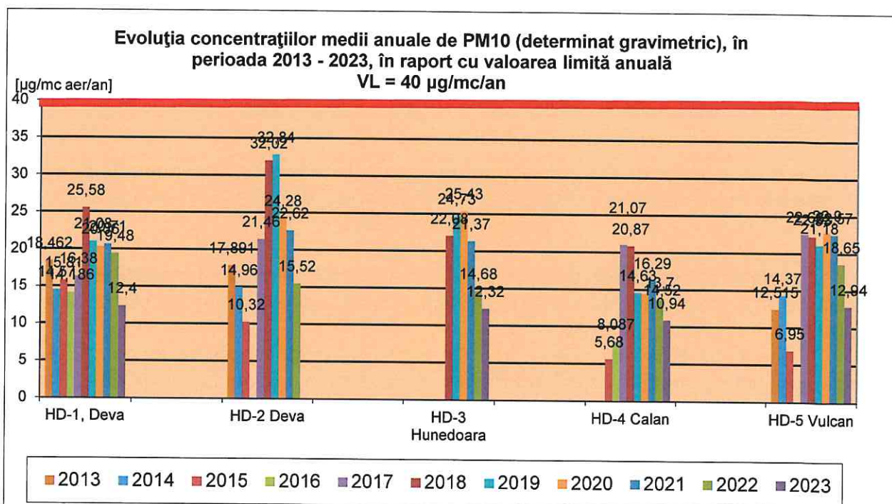
Figura nr. 2.8.3. Evoluția valorilor medii anuale ale PM 10 determinate gravimetric, obținute prin rețeaua automată de monitorizare a calității aerului din județul Hunedoara, în perioada 2013 – 2023
