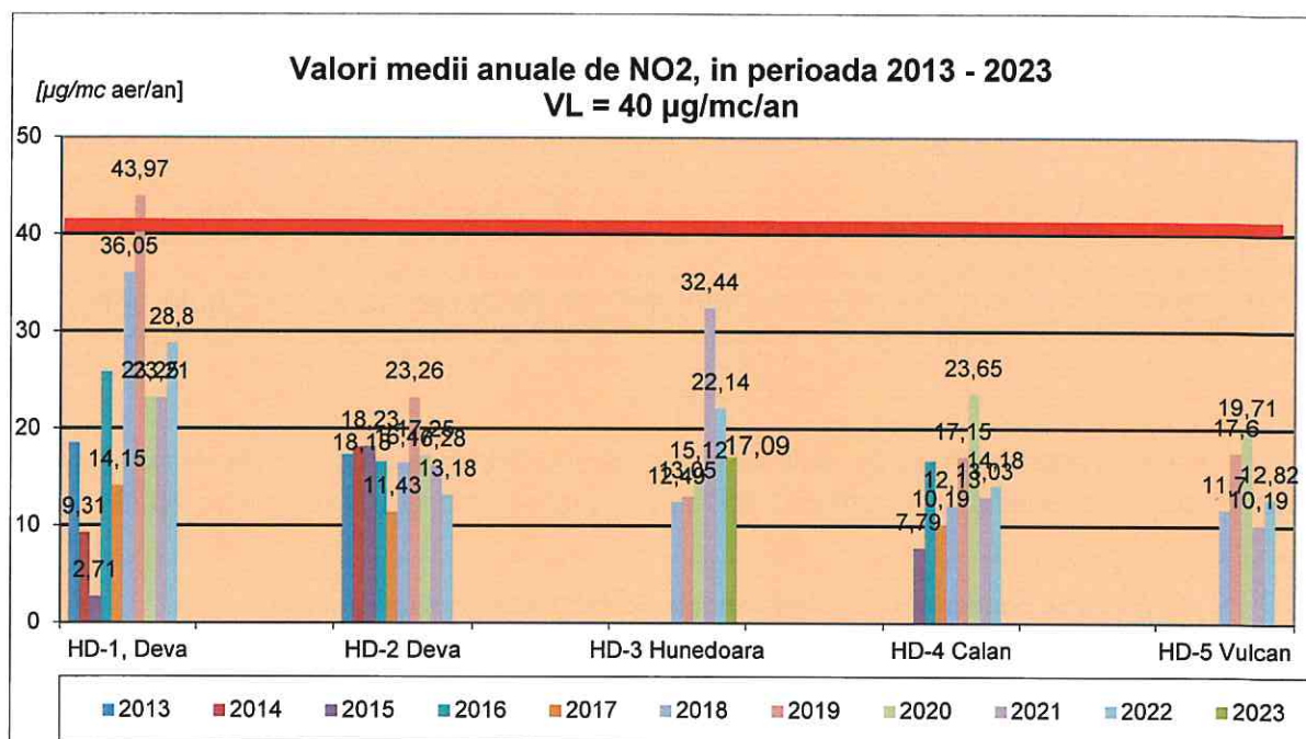
Figura nr. 2.8.1. Evoluția valorilor medii anuale de dioxid de azot obținute prin rețeaua automată de monitorizare a calității aerului din județul Hunedoara, în perioada 2013 – 2023
