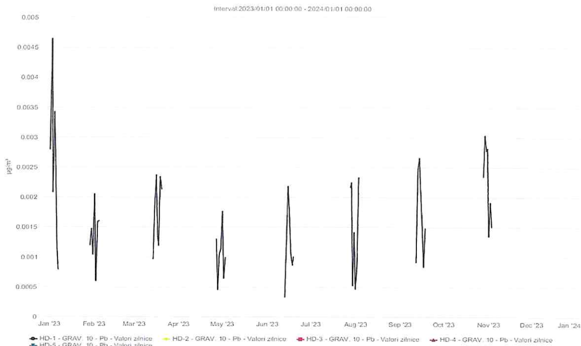
Figura nr. 2.4.1. Evoluția valorilor zilnice de Pb ( \mu\text{g}/\text{mc} ) din PM 10 gravimetric, pe parcursul a 8 săptămâni distribuite uniform pe toată durata anului 2023, la stația automată de monitorizare HD-1 din județul Hunedoara
