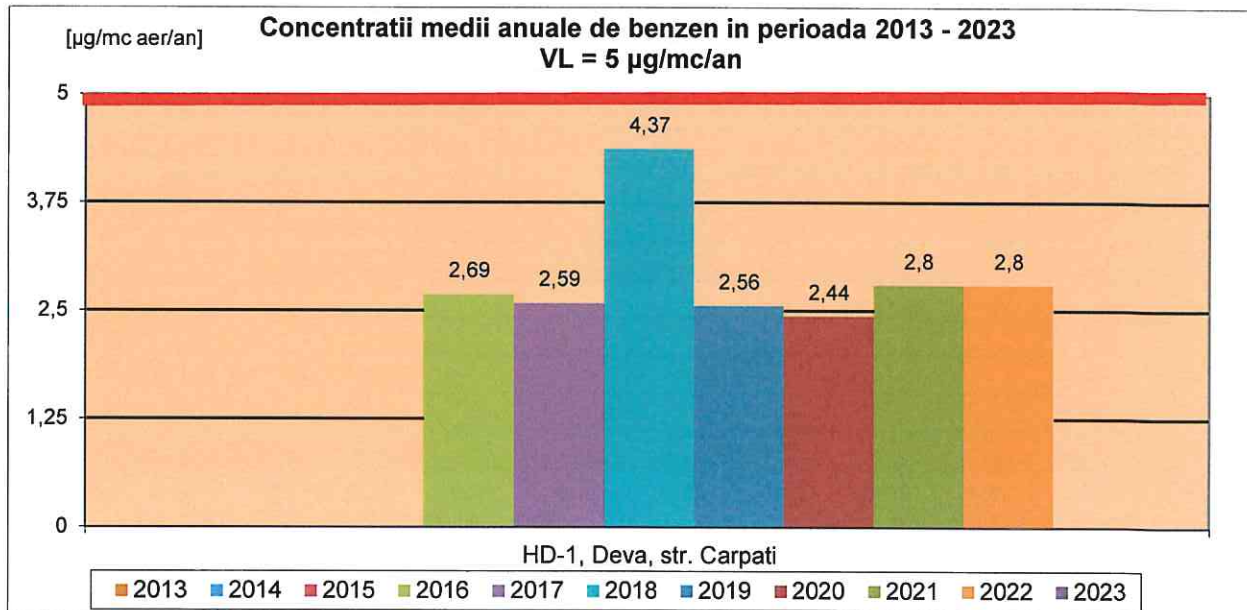
Figura nr. 2.8.5. Evoluția concentrațiilor medii anuale a benzenului, obținută prin rețeaua automată de monitorizare a calității aerului din județul Hunedoara, în perioada 2013 – 2023*
