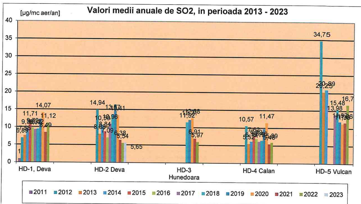
Figura nr. 2.8.2. Evoluția valorilor medii anuale de dioxid de sulf obținute prin rețeaua automată de monitorizare a calității aerului din județul Hunedoara, în perioada 2013– 2023
