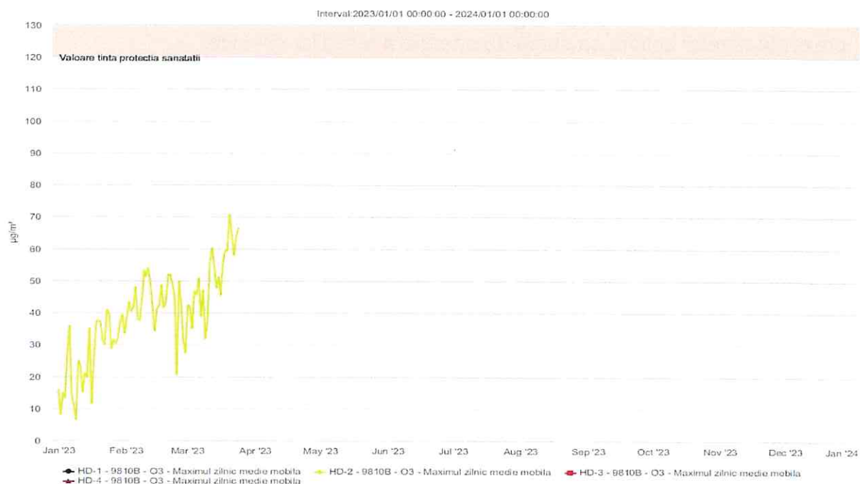
Figura nr. 2.7.2. Evoluția valorilor maxime zilnice a mediilor pe 8 h la ozon ( \mu\text{g}/\text{mc} ) în anul 2023 la stațiile automate de monitorizare din județul Hunedoara
