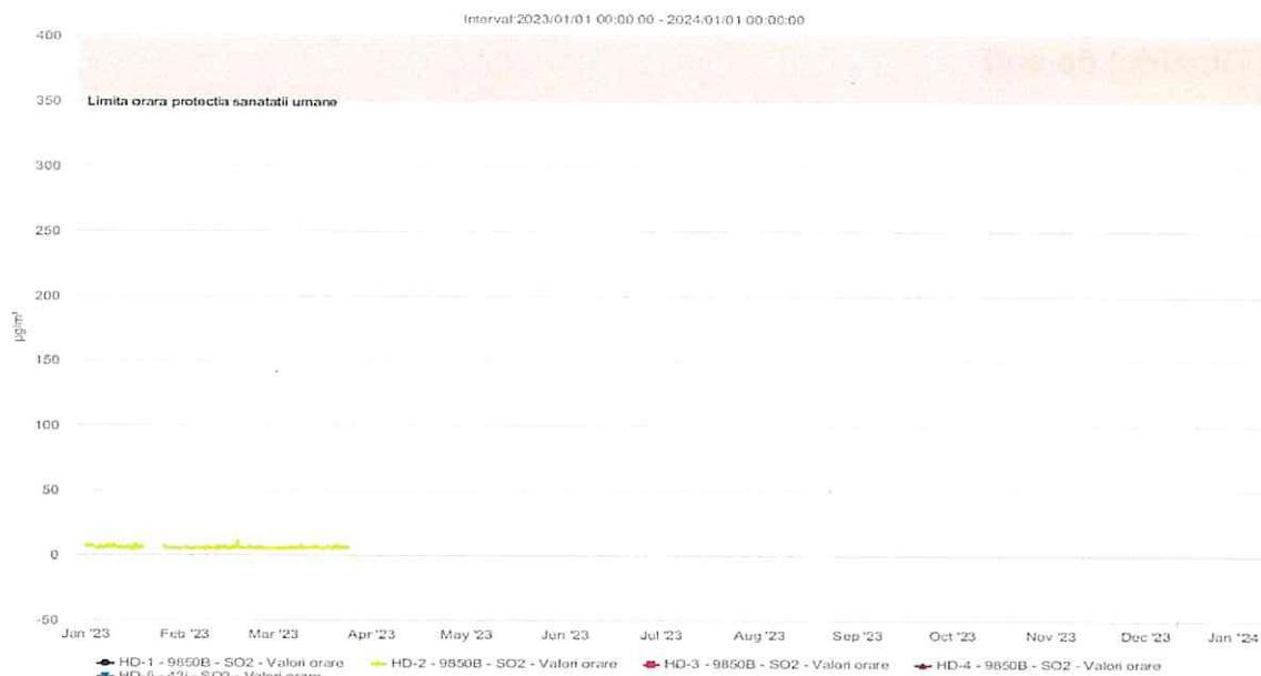
Figura nr. 2.2. 1. Evoluția valorilor orare de SO 2 (µg/mc) în anul 2023, la stațiile automate de monitorizare din județul Hunedoara
