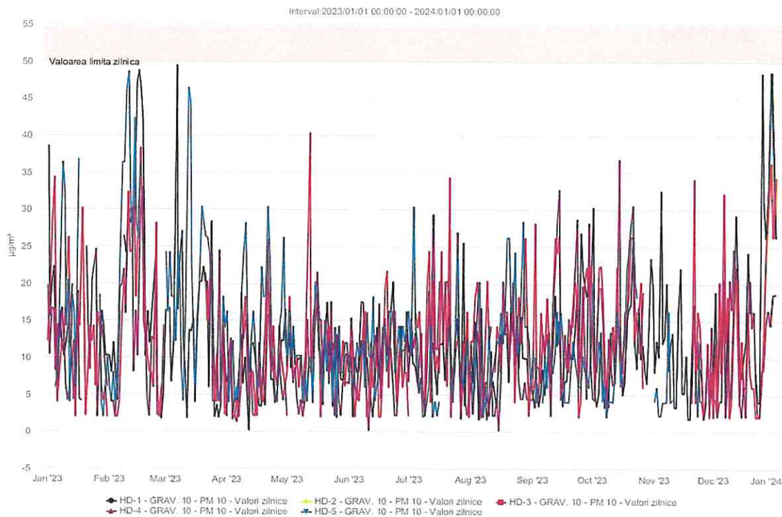
Figura nr. 2.3.2. Evoluția zilnică a valorilor de PM 10 (µg/mc) determinat gravimetric în anul 2023 la stațiile automate de monitorizare din județul Hunedoara
