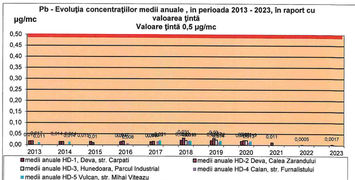
Figura nr. 2.8.7. Evoluția concentrațiilor medii anuale de Pb înregistrate la stațiile automate de monitorizare a calității aerului, în perioada 2013 – 2023, în raport cu valoarea țintă
