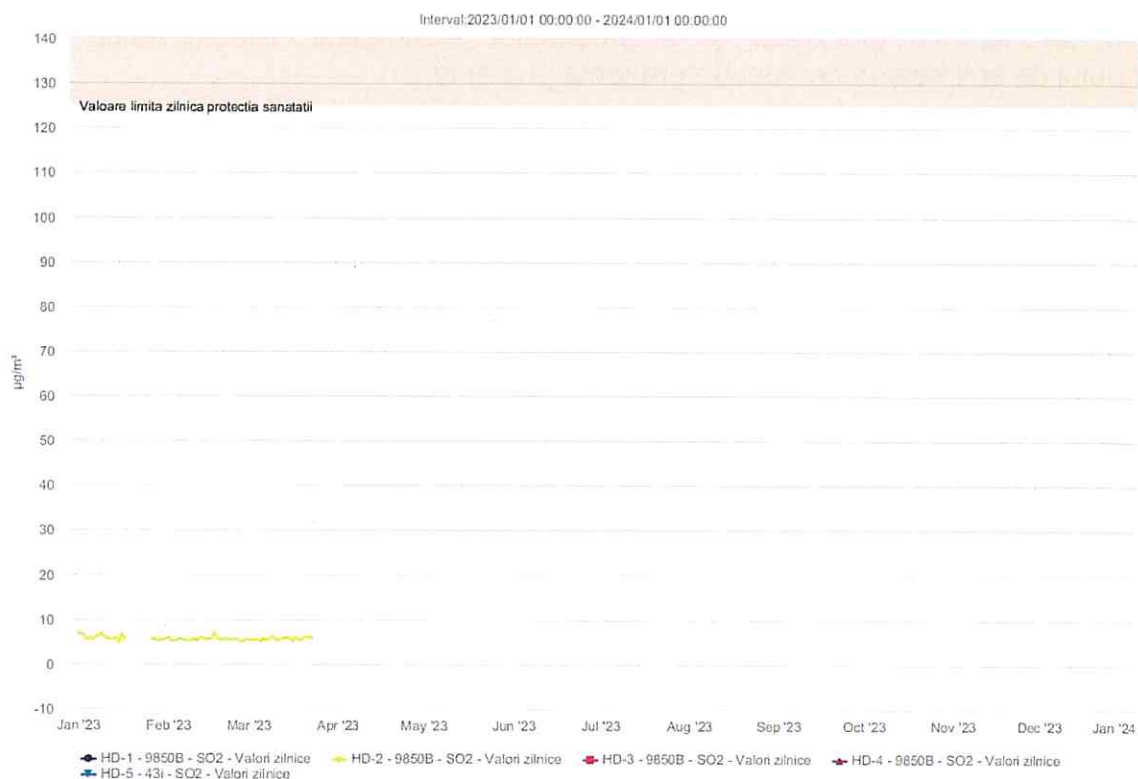
Figura nr. 2.2.2. Evoluția valorilor zilnice de SO 2 (µg/mc) în anul 2023 la stațiile automate de monitorizare din județul Hunedoara
