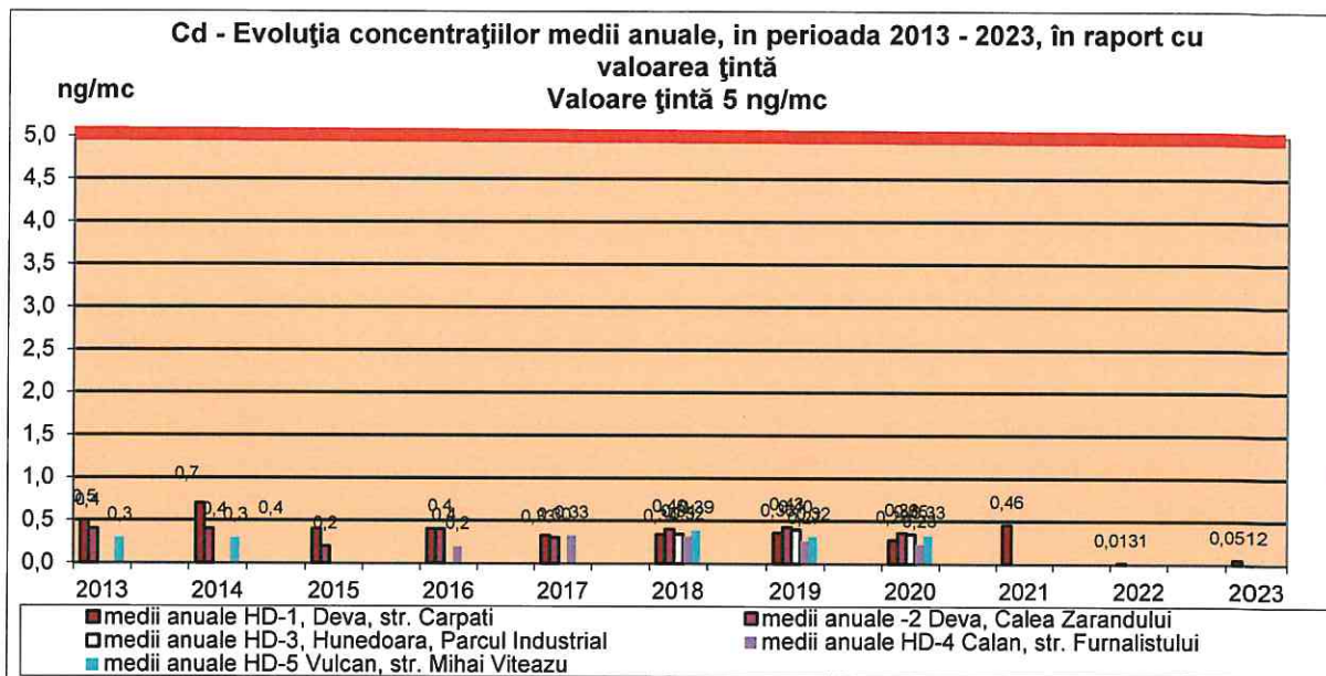
Figura nr. 2.8.8. Evoluția concentrațiilor medii anuale de Cd înregistrate la stațiile automate de monitorizare a calității aerului, în perioada 2013 – 2023, în raport cu valoarea țintă
