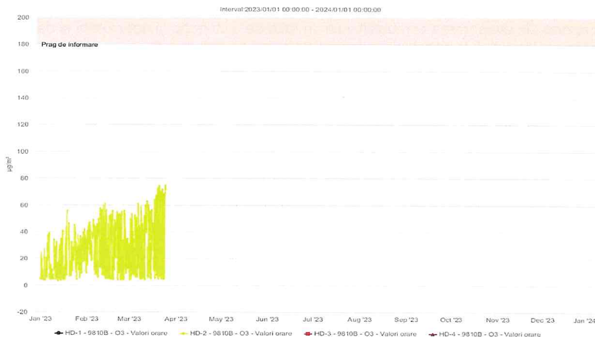
Figura nr. 2.7.1. Evoluția valorilor orare la ozon ( \mu\text{g}/\text{mc} ) în anul 2023 la stațiile automate de monitorizare din județul Hunedoara
