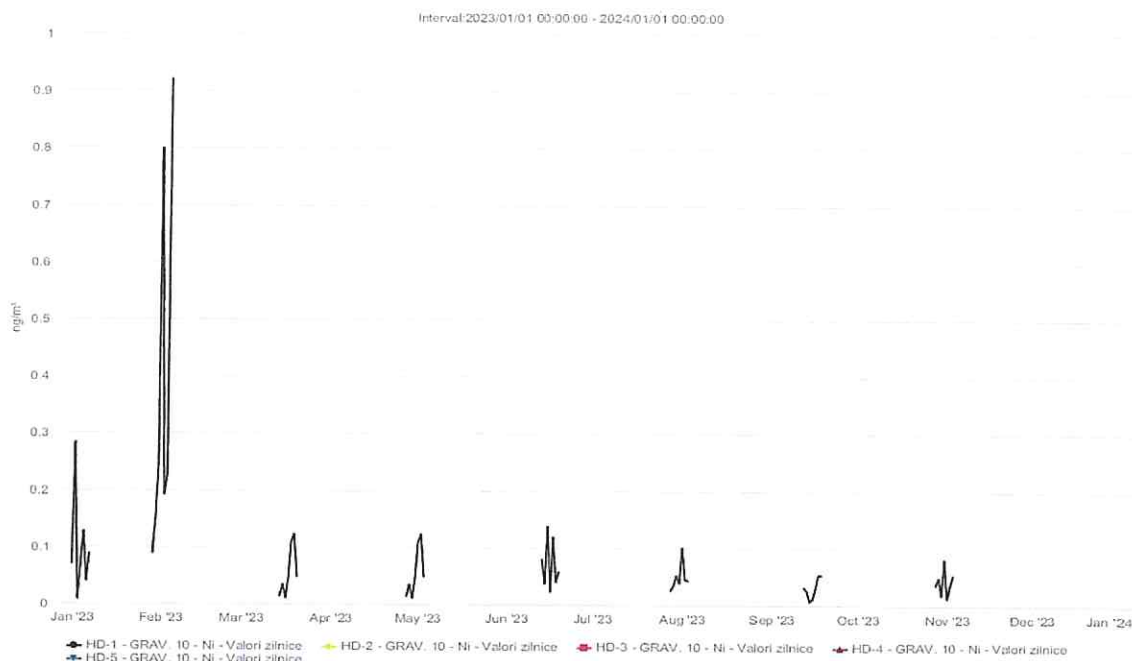
Figura nr. 2.4.3. Evoluția valorilor zilnice de Ni (ng/mc) din PM 10 gravimetric, pe parcursul a 8 săptămâni distribuite uniform pe toată durata anului 2023, la stația automată de monitorizare HD-1 din județul Hunedoara
