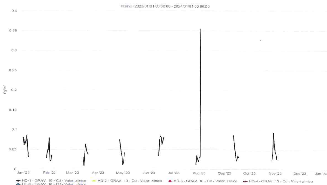
Figura nr. 2.4.2. Evoluția valorilor zilnice de Cd ( \text{ng}/\text{mc} ) din PM 10 gravimetric, pe parcursul a 8 săptămâni distribuite uniform pe toată durata anului 2023, la stația automată de monitorizare HD-1 din județul Hunedoara
