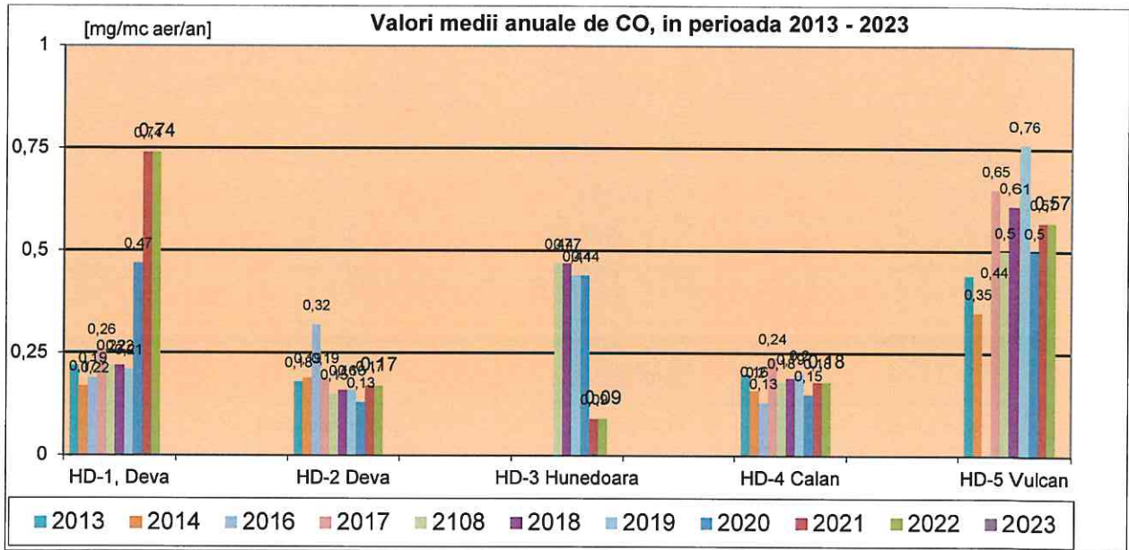
Figura nr. 2.8.4. Evoluția valorilor medii anuale de monoxid de carbon obținute prin rețeaua automată de monitorizare a calității aerului din județul Hunedoara, în perioada 2013 – 2023*
