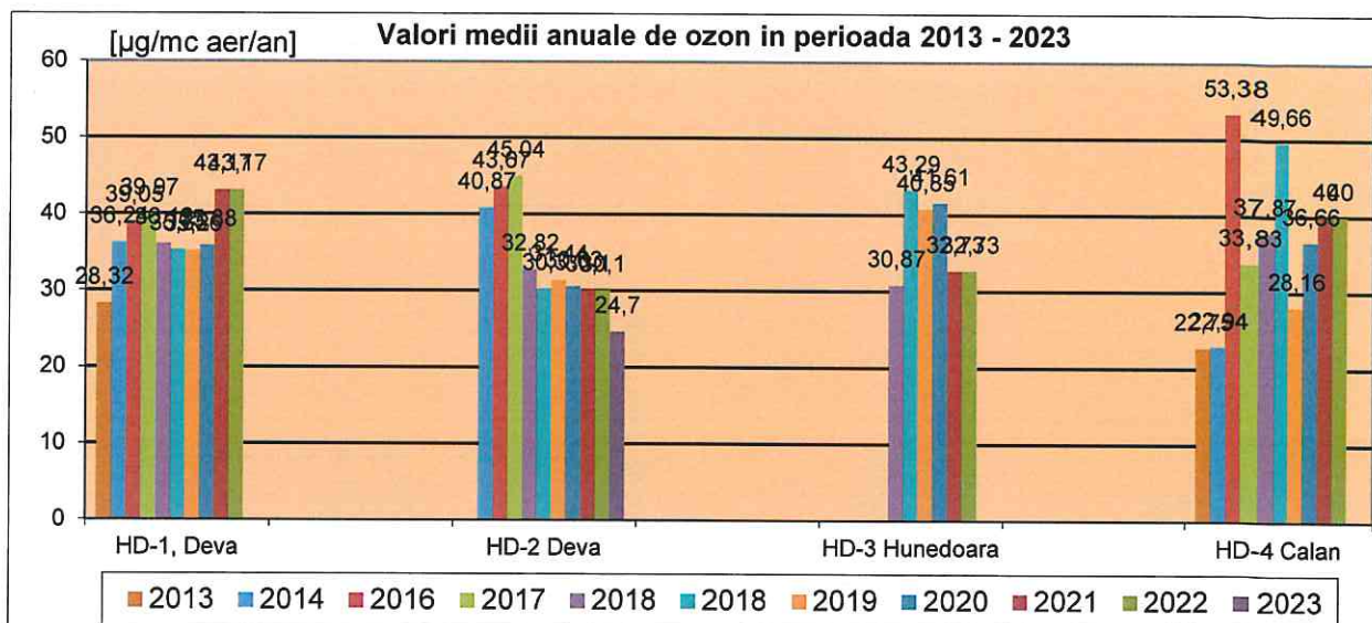
Figura nr. 2.8.6. Evoluția valorilor medii anuale ale ozonului, obținute prin rețeaua automată de monitorizare a calității aerului din județul Hunedoara, în perioada 2013 – 2023
