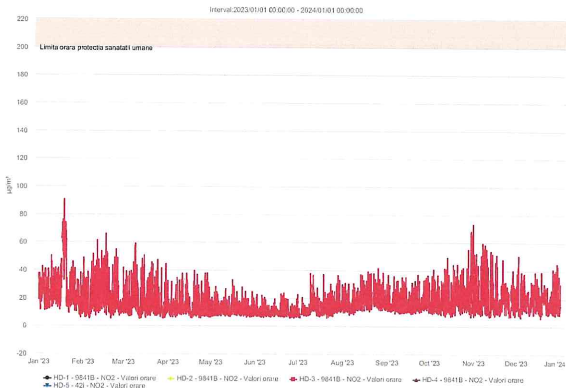
Figura nr. 2 1.1. Evoluția valorilor orare de NO 2 (μg/mc), în anul 2023, la stațiile automate de monitorizare din județul Hunedoara
