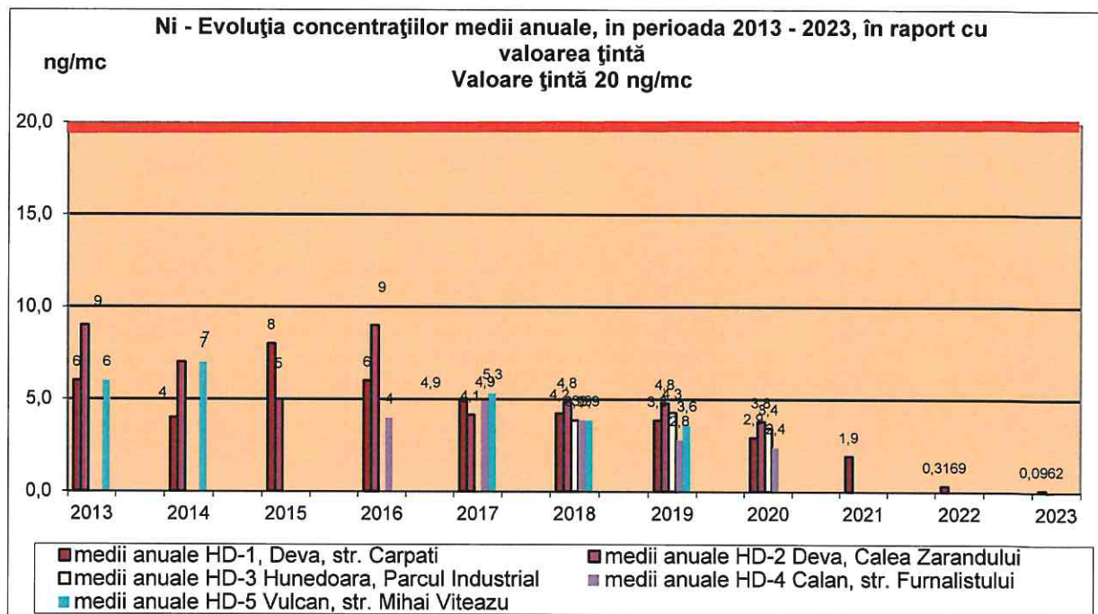
Figura nr. 2.8.9. de monitorizare a calității aerului, în perioada 2013 – 2023, în raport cu valoarea țintă
