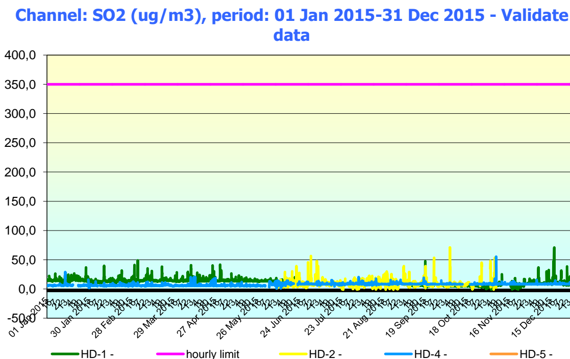
Figura nr. 2.2.1. Evoluția valorilor orare de \text{SO}_2 ( \mu\text{g}/\text{mc} ) în anul 2015, la stațiile automate de monitorizare
