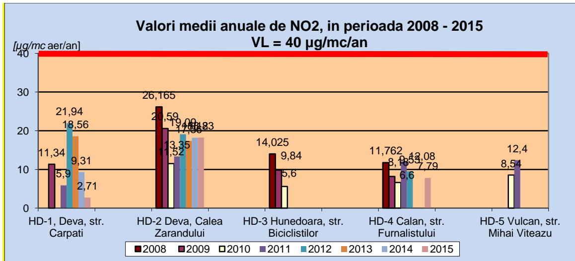
Figura nr. 2.8.1. Evoluția valorilor medii anuale de dioxid de azot obținute prin rețeaua automată de monitorizare a calității aerului, în perioada 2008 - 2015
