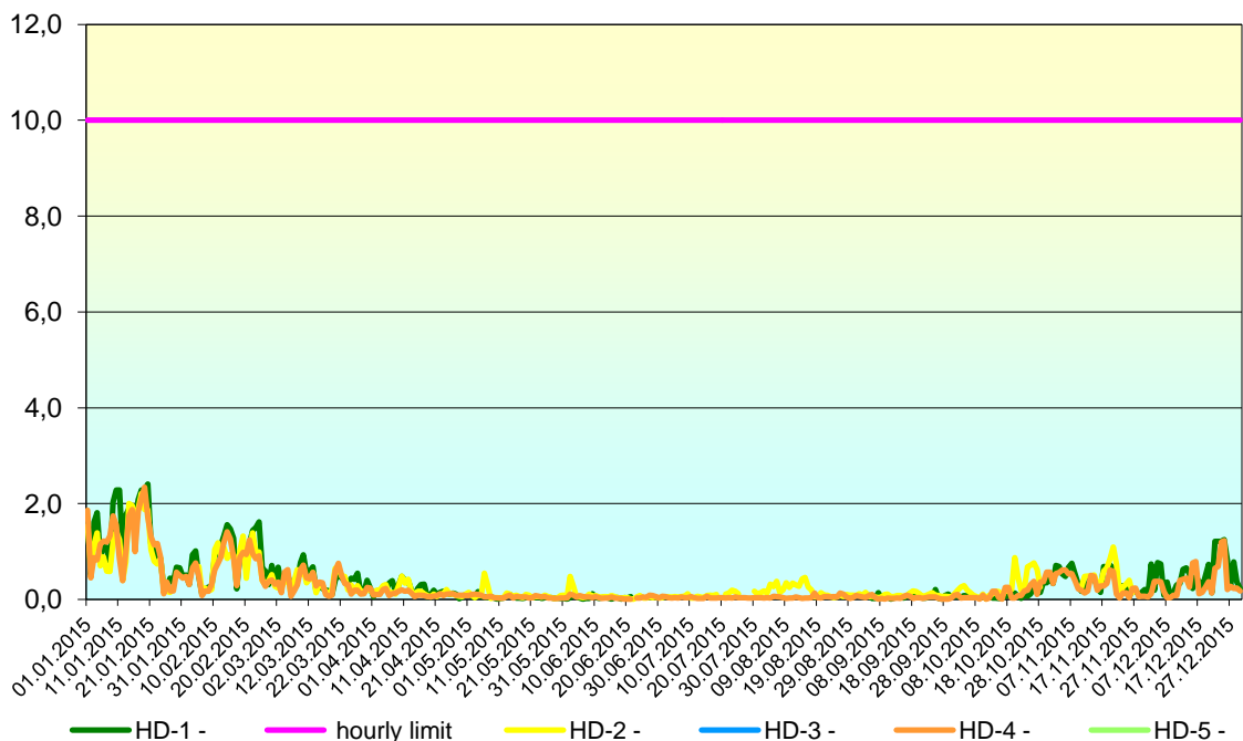
Figura nr. 2.5.1. Evoluția valorilor maxime zilnice a mediilor pe 8h de CO (mg/mc) în anul 2015 la stațiile automate de monitorizare
