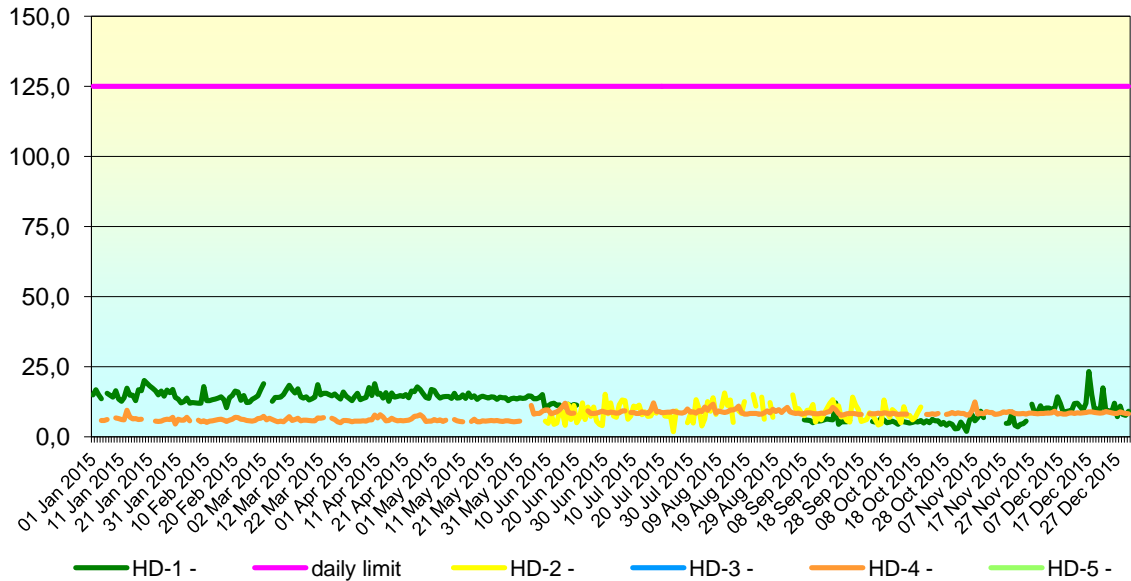
Figura nr. 2.2.2. Evoluția valorilor zilnice de SO 2 (ug/mc) în anul 2015, la stațiile automate de monitorizare
