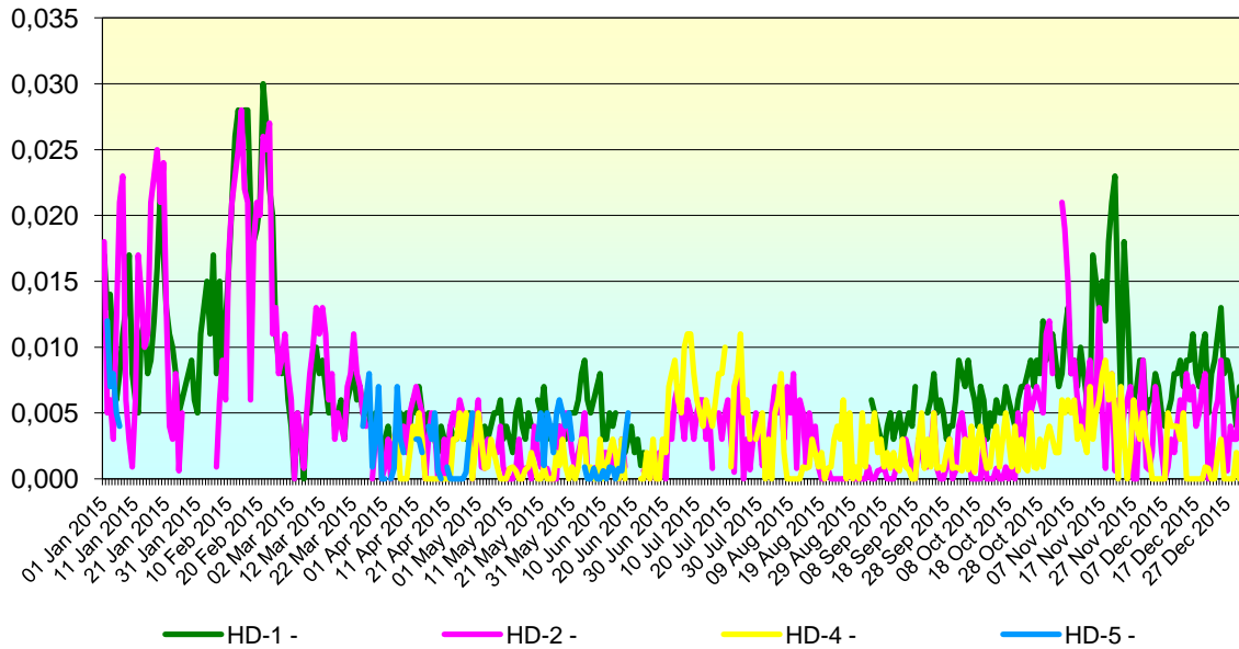
Figura nr. 2.4.3. Evoluția valorilor zilnice de Ni ( \mu\text{g}/\text{mc} ) din PM 10 gravimetric în anul 2015, la stațiile automate de monitorizare
