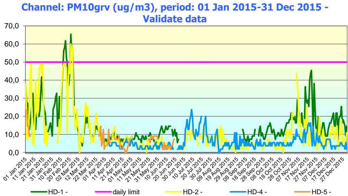
Figura nr. 2.3.2. Evoluția zilnică a valorilor de PM 10 (μg/mc) determinat gravimetric în anul 2015, la stațiile automate de monitorizare
