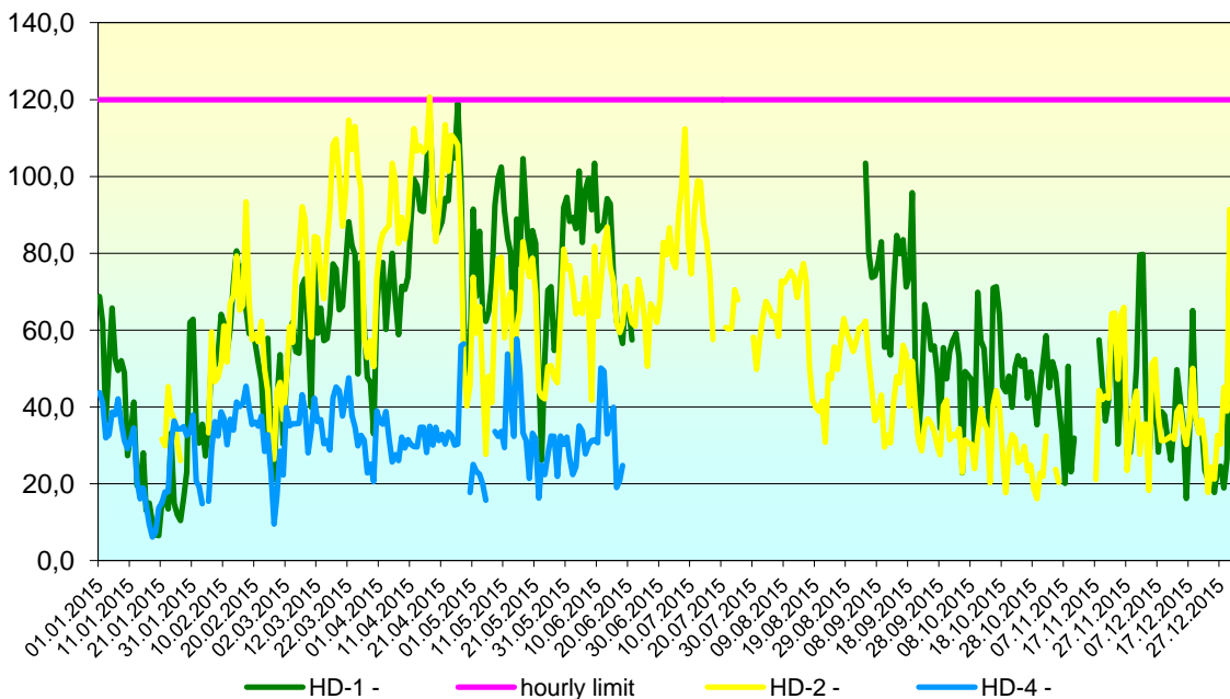
Figura nr. 2.7.2. Evoluția valorilor maxime zilnice a mediilor pe 8 h la ozon (µg/mc) în anul 2015 la stațiile automate de monitorizare
