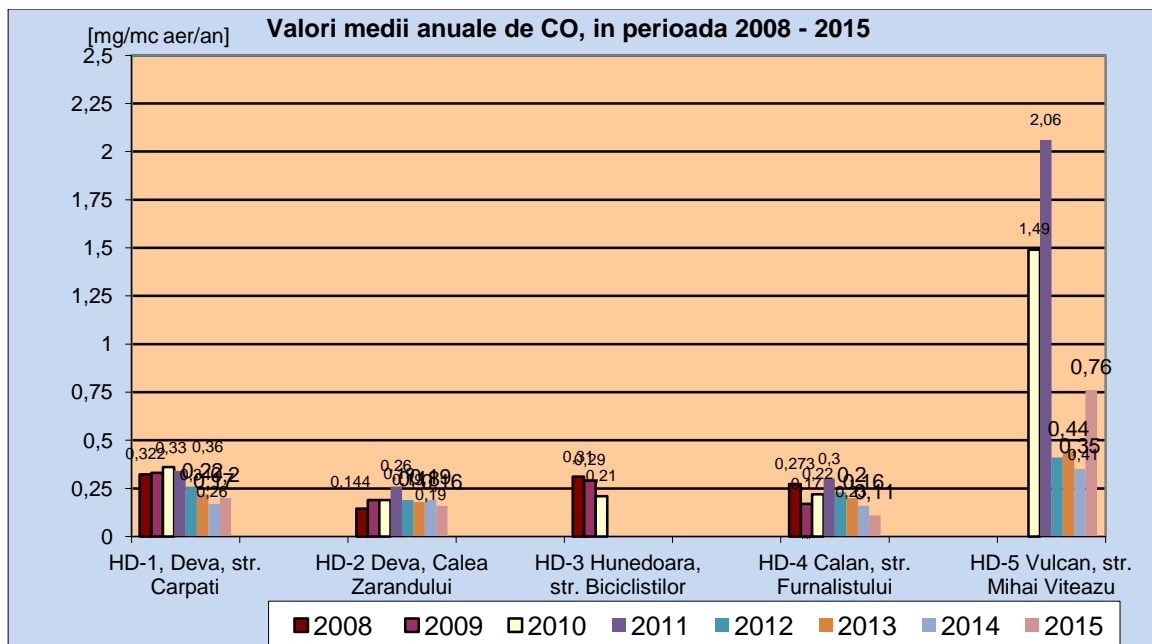
Figura nr. 2.8.5. Evoluția valorilor medii anuale de monoxid de carbon obținute prin rețeaua automată de monitorizare a calității aerului, în perioada 2008 – 2015
