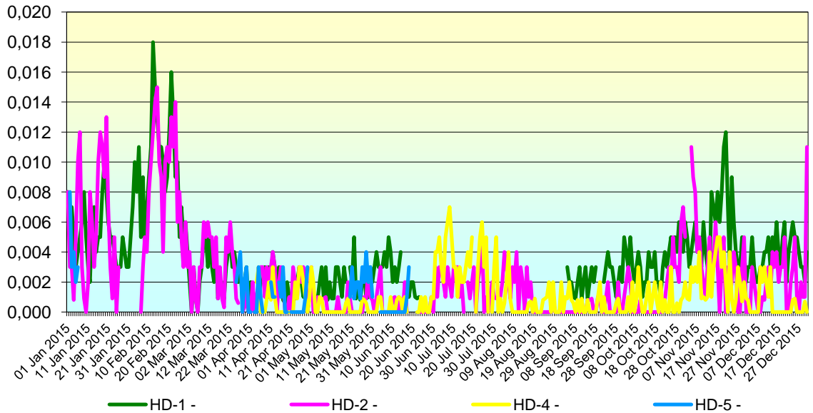
Figura nr. 2.4.2. Evoluția valorilor zilnice de Cd ( \mu\text{g}/\text{mc} ) din PM 10 gravimetric în anul 2015, la stațiile automate de monitorizare
