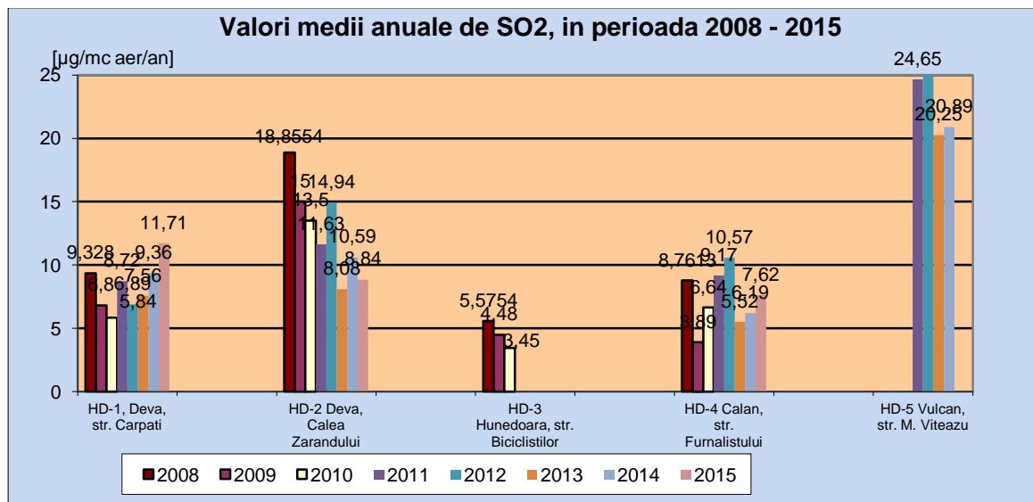
Figura nr. 2.8.2. Evoluția valorilor medii anuale de dioxid de sulf obținute prin rețeaua automată de monitorizare a calității aerului, în perioada 2008 – 2015
