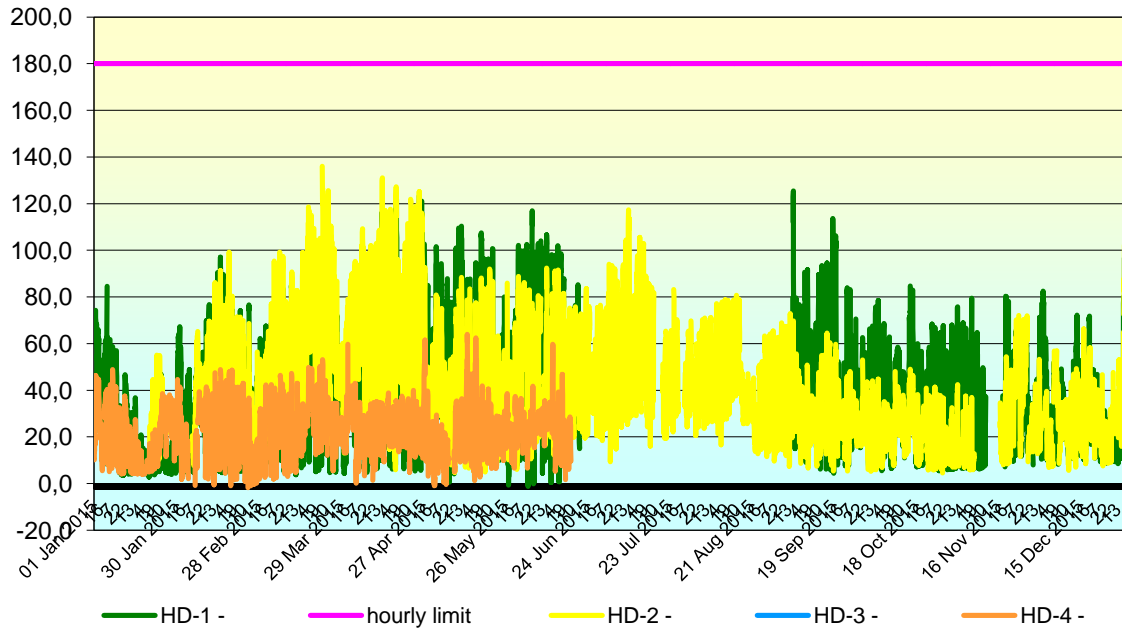
Figura nr. 2.7.1. Evoluția valorilor zilnice la ozon (µg/mc) în anul 2015 la stațiile automate de monitorizare
