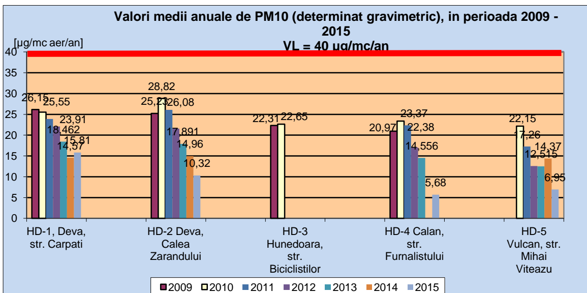
Figura nr. 2.8.4. Evoluția valorilor medii anuale ale PM 10 determinate gravimetric, obținute prin rețeaua automată de monitorizare a calității aerului, în perioada 2009 – 2015
