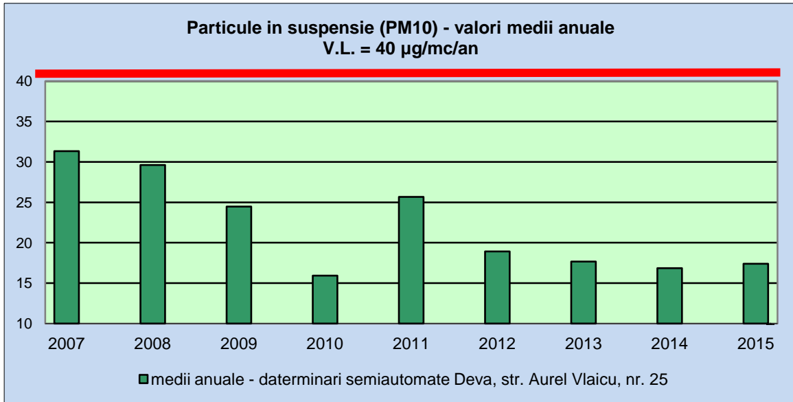
Fig. 2.8.3 Evoluția particulelor în suspensie (PM 10 ), în perioada 2007 – 2015, obținute prin determinări semiautomate la punctul situat în Deva, str. Aurel Vlaicu, nr.25
