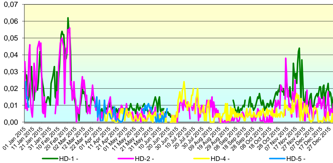
Figura nr. 2.4.1. Evoluția valorilor zilnice de Pb ( \mu\text{g}/\text{mc} ) din PM 10 gravimetric în anul 2015, la stațiile automate de monitorizare
