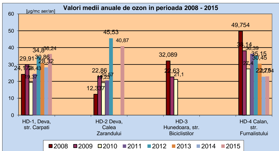
Figura nr. 2.8.6. Evoluția valorilor medii anuale ale ozonului, obținute prin rețeaua automată de monitorizare a calității aerului în perioada 2008-2015
