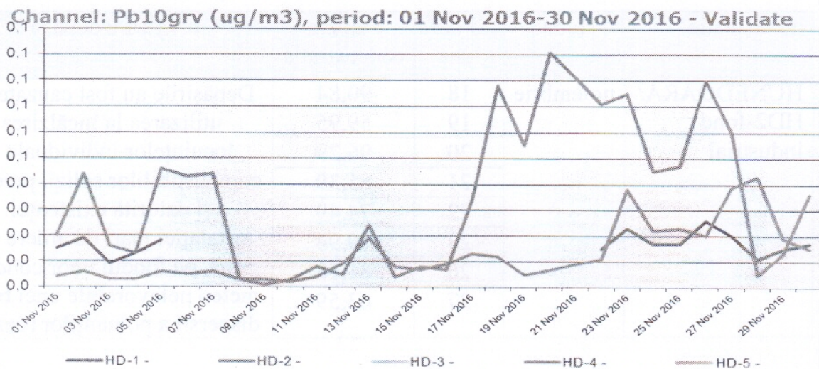
Figura nr. 1.3.8. Evoluția valorilor zilnice de Pb ( \mu\text{g}/\text{mc} ) din PM_{10} gravimetric, în luna noiembrie 2016, la stațiile automate de monitorizare
