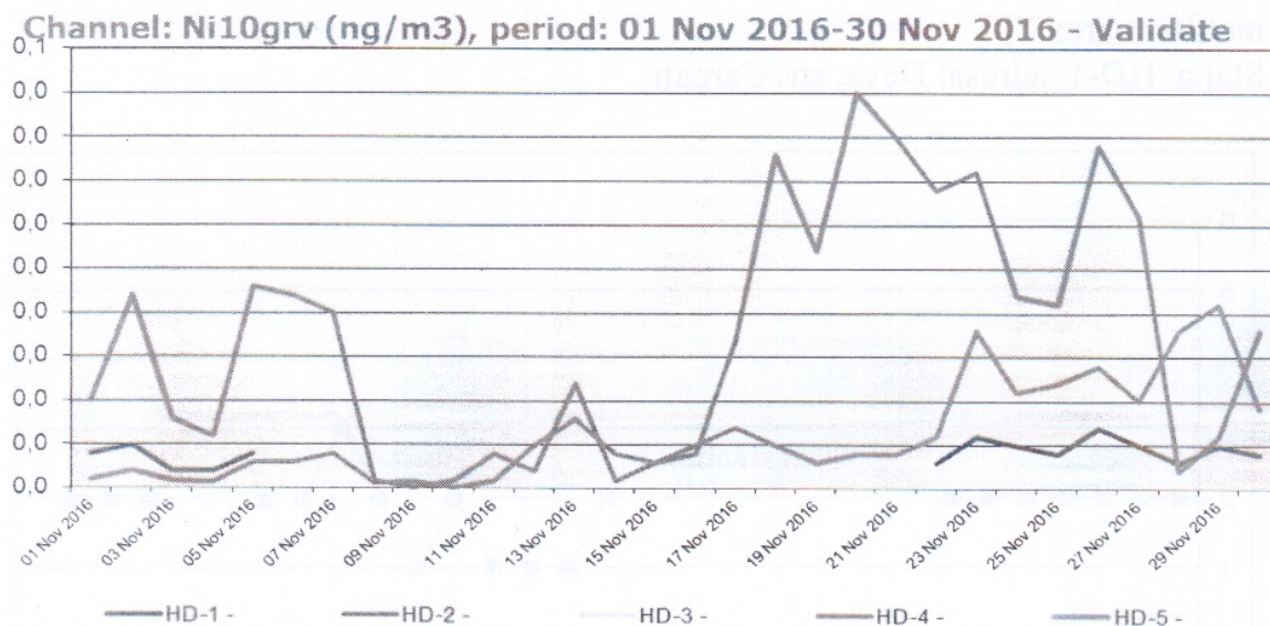
Figura nr.1.3.10. Evoluția valorilor zilnice de Ni ( \mu\text{g}/\text{mc} ) din \text{PM}_{10} gravimetric, în luna noiembrie 2016, la stațiile automate de monitorizare
