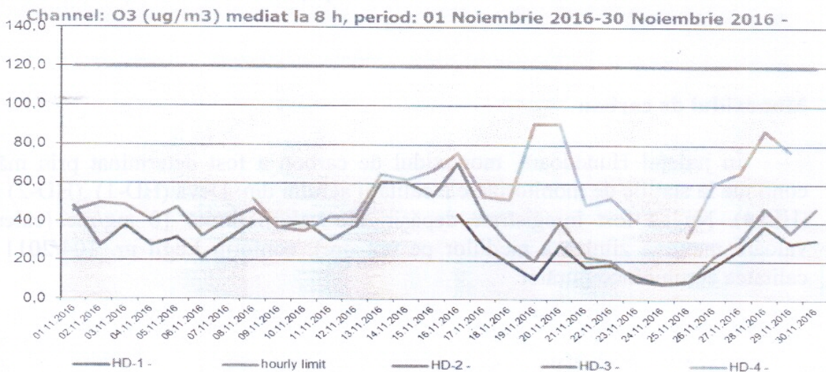
Figura nr. 1.3.6. Evoluția valorilor maxime zilnice a mediilor pe 8 ore la ozon ( \mu\text{g}/\text{mc} ), în luna noiembrie 2016, la stațiile automate de monitorizare
