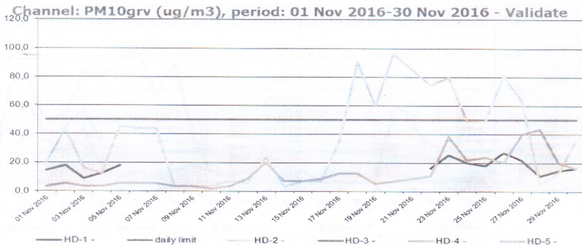
Figura nr. 1.3.7. Evoluția zilnică a valorilor de PM 10 (μg/mc) determinat gravimetric, în luna noiembrie 2016, la stațiile automate de monitorizare
