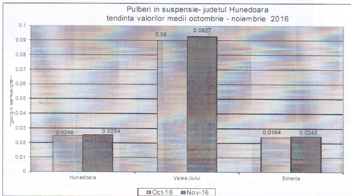
Fig. nr. 1.2.1.1. Evoluția calității pulberilor în suspensie în perioada octombrie – noiembrie 2016
