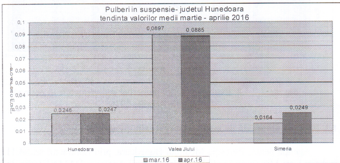
Fig. nr. 1.2.1.1. Evoluția calității pulberilor în suspensie în perioada martie – aprilie 2016
