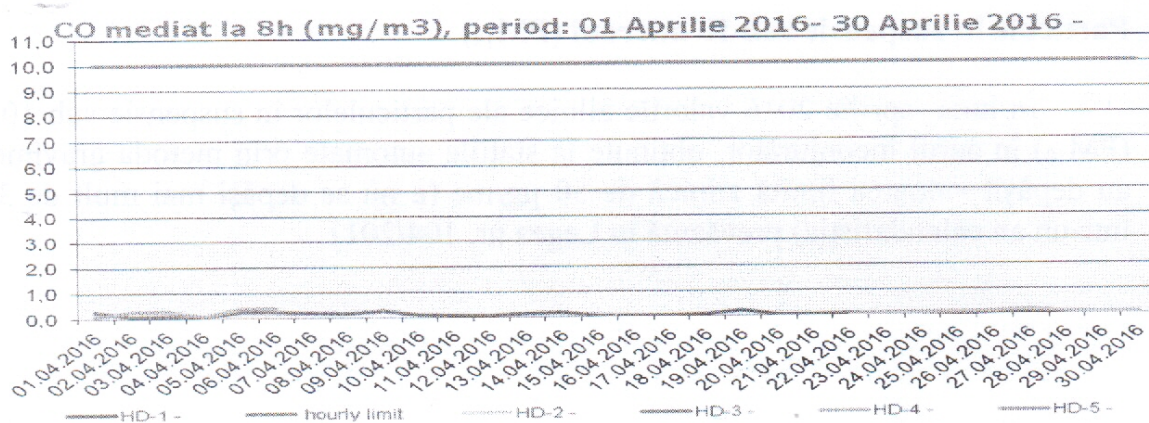
Figura nr. 1.3.5. Evoluția valorilor maxime zilnice a mediilor pe 8 ore la CO ( \text{mg}/\text{mc} ), în luna aprilie 2016, la stațiile automate de monitorizare
