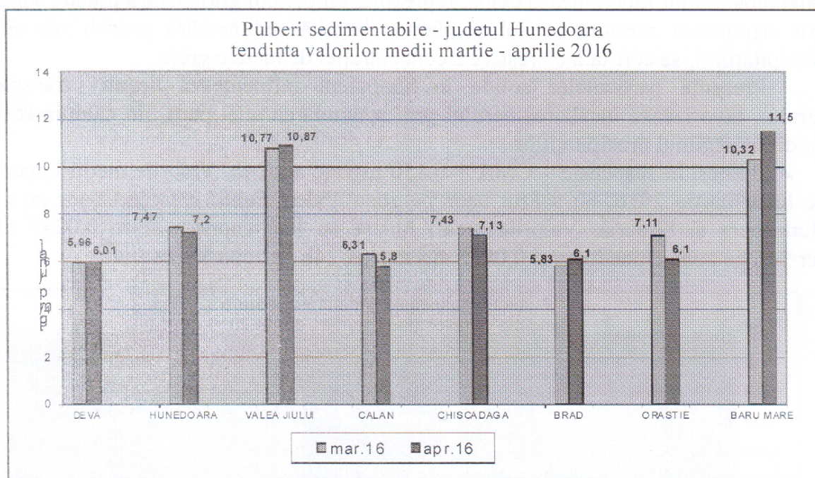
Fig. nr. 1.2.1.2. Evoluția calității pulberilor sedimentabile în perioada martie - aprilie 2016
