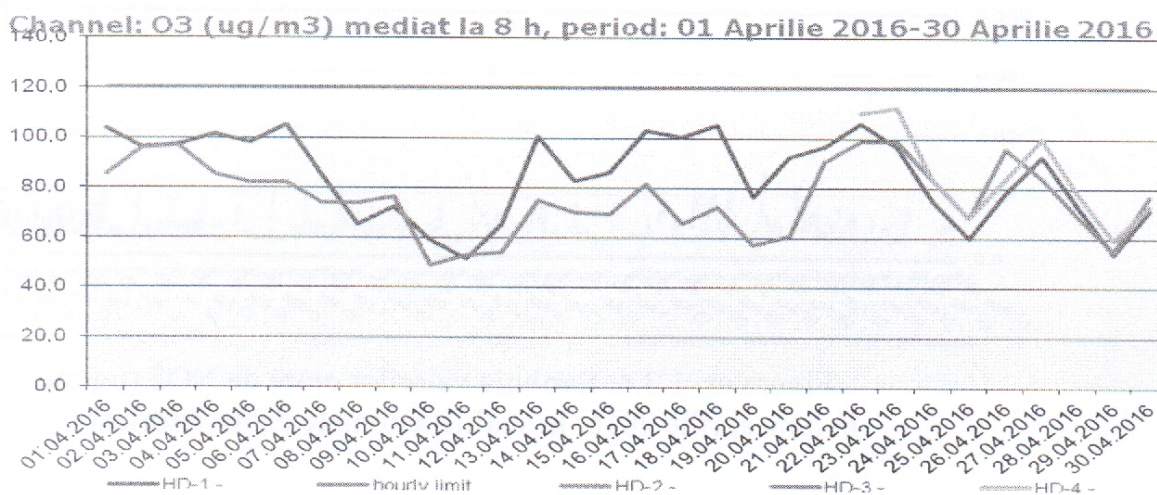
Figura nr. 1.3.6. Evoluția valorilor maxime zilnice a mediilor pe 8 ore la ozon ( \mu\text{g}/\text{mc} ), în luna aprilie 2016, la stațiile automate de monitorizare
