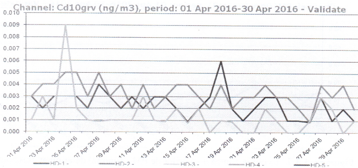
Figura nr. 1.3.9. Evoluția valorilor zilnice de Cd ( \mu\text{g}/\text{mc} ) din \text{PM}_{10} gravimetric, în luna aprilie 2016, la stațiile automate de monitorizare
