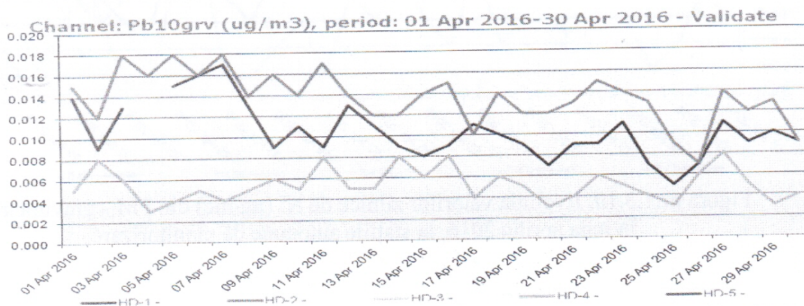
Figura nr. 1.3.8. Evoluția valorilor zilnice de Pb (µg/mc) din PM 10 gravimetric, în luna aprilie 2016, la stațiile automate de monitorizare
