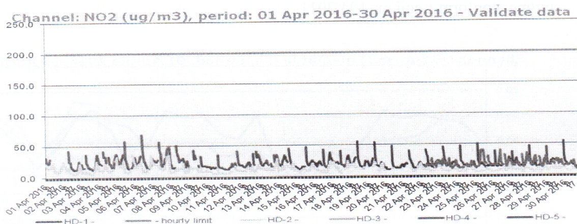
Figura nr. 1.3.4. Evoluția valorilor orare de NO 2 ( \mu\text{g}/\text{mc} ), în luna aprilie 2016, la stațiile automate de monitorizare
