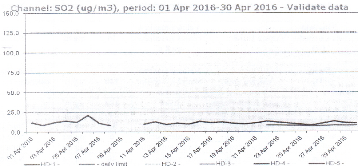
Figura nr. 1.3.3. Evoluția valorilor zilnice de SO2 ( \mu\text{g}/\text{mc} ), în luna aprilie 2016, la stațiile automate de monitorizare
