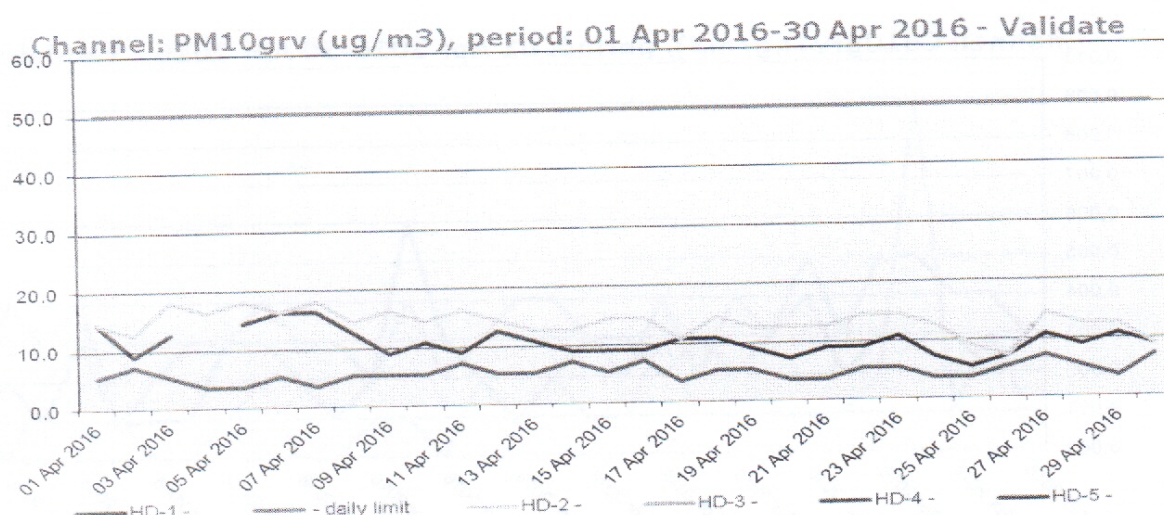
Figura nr. 1.3.7. Evoluția zilnică a valorilor de PM 10 (µg/mc) determinat gravimetric, în luna aprilie 2016, la stațiile automate de monitorizare
