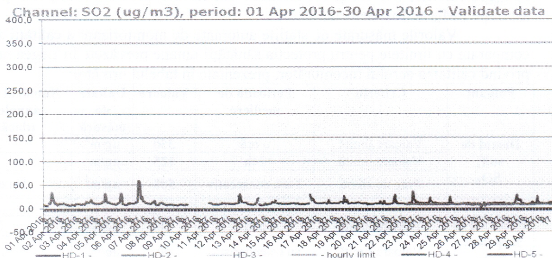
Figura nr. 1.3.2. Evoluția valorilor orare de SO2 ( \mu\text{g}/\text{mc} ), în luna aprilie 2016, la stațiile automate de monitorizare
