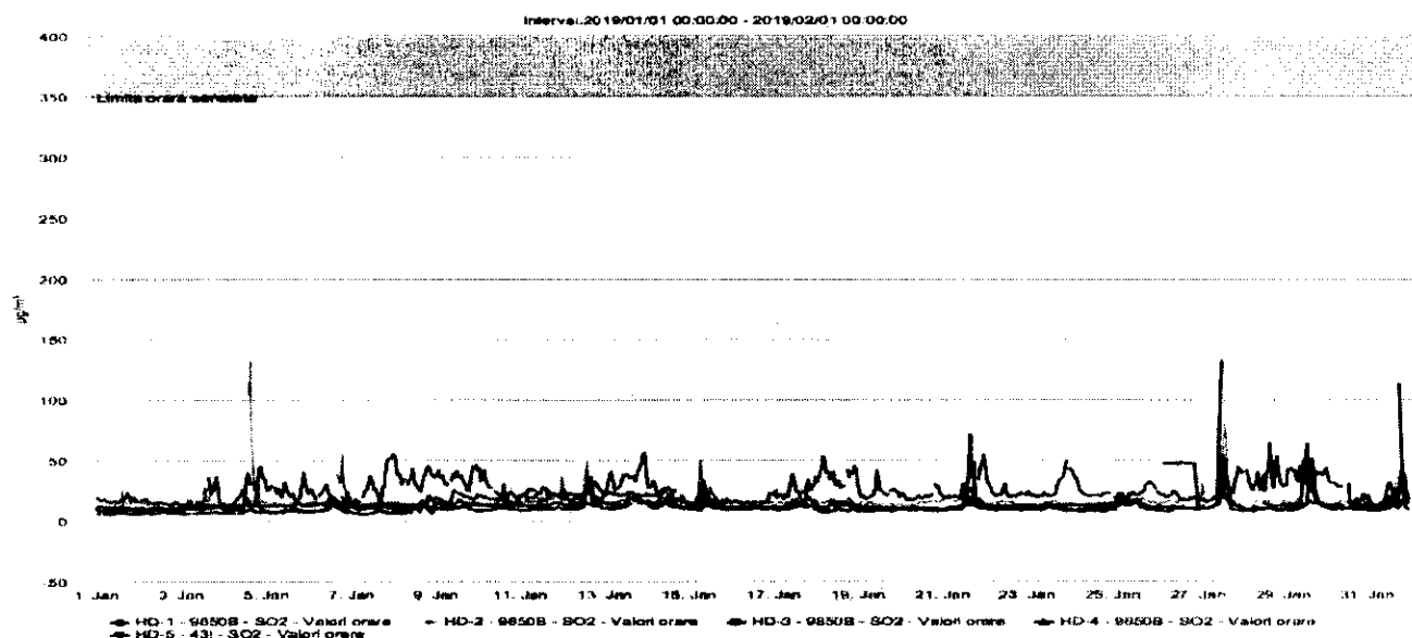
Figura nr. 1.3.2. Evoluția valorilor orare de SO 2 ( \mu\text{g}/\text{mc} ), în luna ianuarie 2019 la stațiile automate de monitorizare
