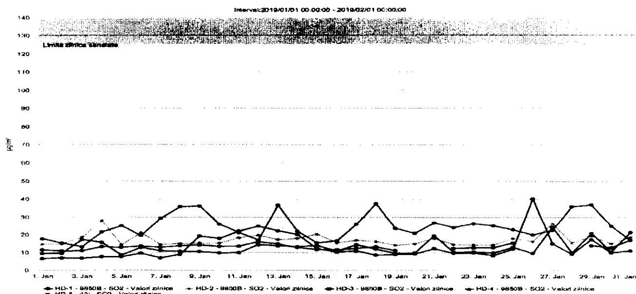
Figura nr. 1.3.3. Evoluția valorilor zilnice de SO 2 ( \mu\text{g}/\text{mc} ), în luna ianuarie 2019, la stațiile automate de monitorizare
