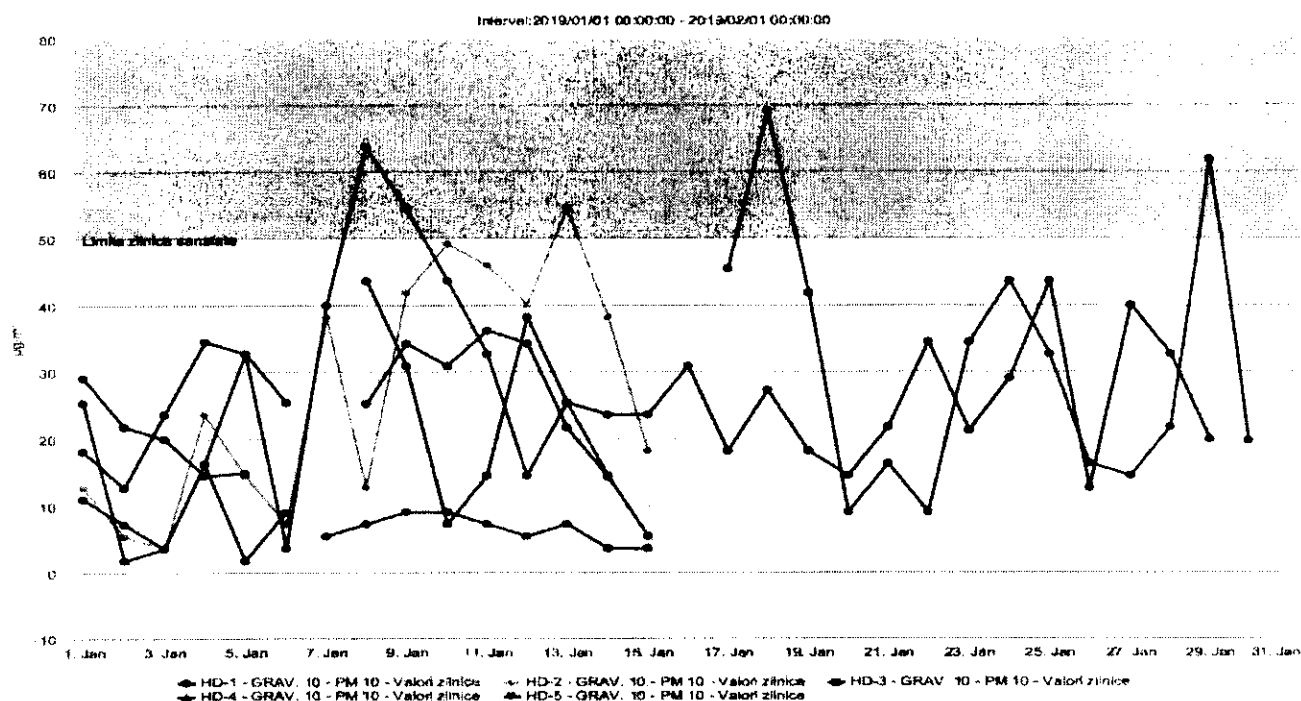
Figura nr. 1.3.7. Evoluția zilnică a valorilor de PM 10 (µg/mc) determinat gravimetric, în luna ianuarie 2019, la stațiile automate de monitorizare
