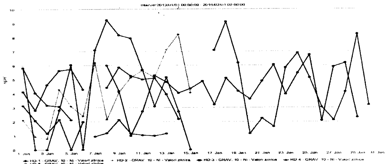
Figura nr.1.3.10. Evoluția valorilor zilnice de Ni ( \mu\text{g}/\text{mc} ) din \text{PM}_{10} gravimetric, în luna ianuarie 2019, la stațiile automate de monitorizare
