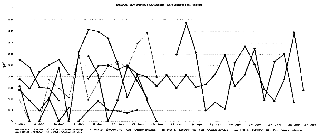
Figura nr. 1.3.9. Evoluția valorilor zilnice de Cd (μg/mc) din PM 10 gravimetric, în luna ianuarie 2019, la stațiile automate de monitorizare
