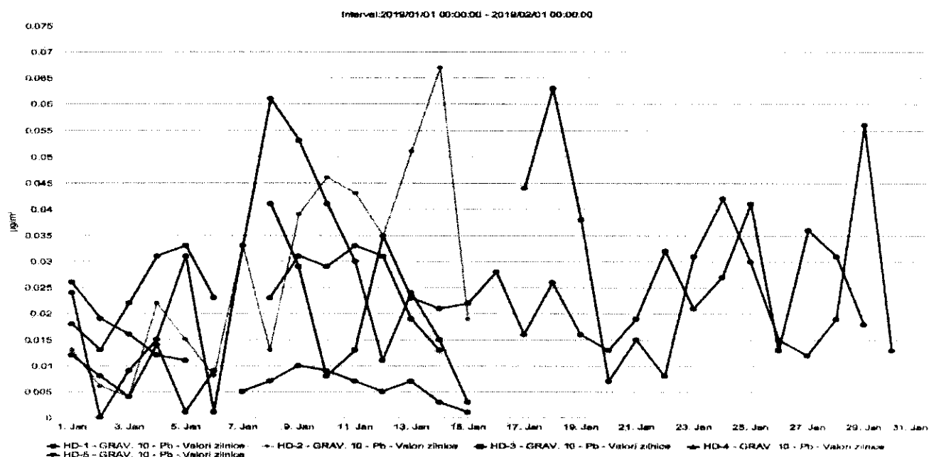
Figura nr. 1.3.8. Evoluția valorilor zilnice de Pb (μg/mc) din PM 10 gravimetric, în luna ianuarie 2019, la stațiile automate de monitorizare
