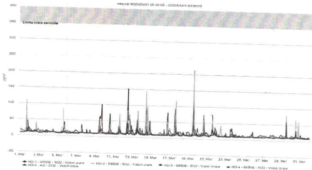
Figura nr. 1.3.2. Evoluția valorilor orare de SO 2 ( \mu\text{g}/\text{mc} ), în luna martie 2020 la stațiile automate de monitorizare
