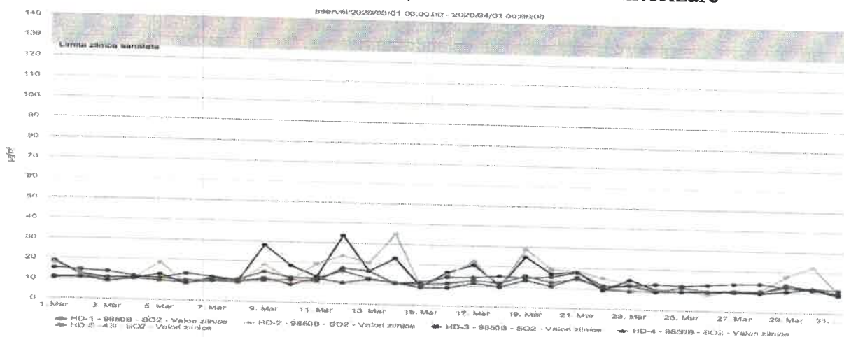
Figura nr. 1.3.2. Evoluția valorilor orare de SO 2 ( \mu\text{g}/\text{mc} ), în luna martie 2020 la stațiile automate de monitorizare
